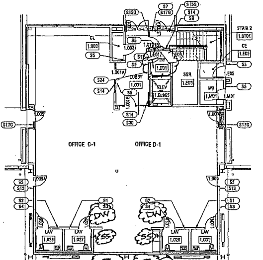
3 Reference Plan - Office Pod 2 - Level 1 A10.11 Scale: 1/8" = 1'-0"
