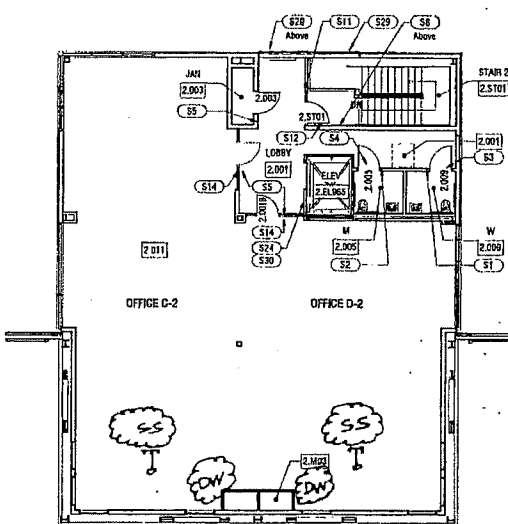
4 Reference Plan - Office Pod 2 - Level 2 A10.11 Scale: 1/8" = 1'-0"
