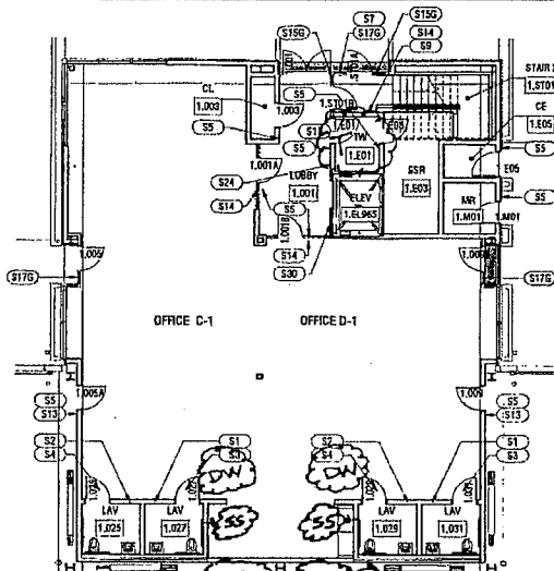
3 Reference Plan - Office Pod 2 - Level 1 A10.11 Scale: 1/8" = 1'-0"
