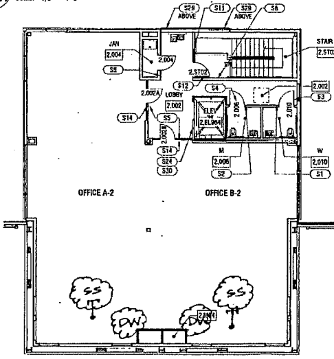
2 Reference Plan - Office Pod 1 - Level 2 A10.11 Scale: 1/8" = 1'-0"
