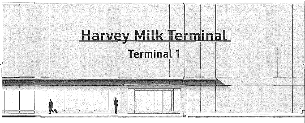
Elevation Scale: 1/8" = 1'-0"
