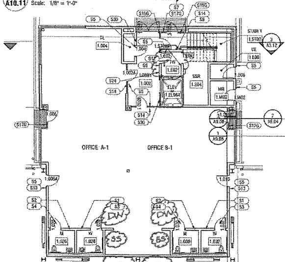
1 Reference Plan - Office Pod 1 - Level 1 A10.11 Scale: 1/8" = 1'-0"
