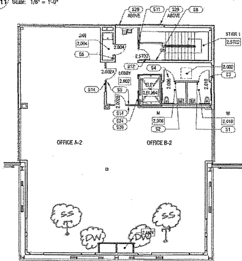
2 Reference Plan - Office Pod 1 - Level 2 A10.11 Scale: 1/8" = 1'-0"
