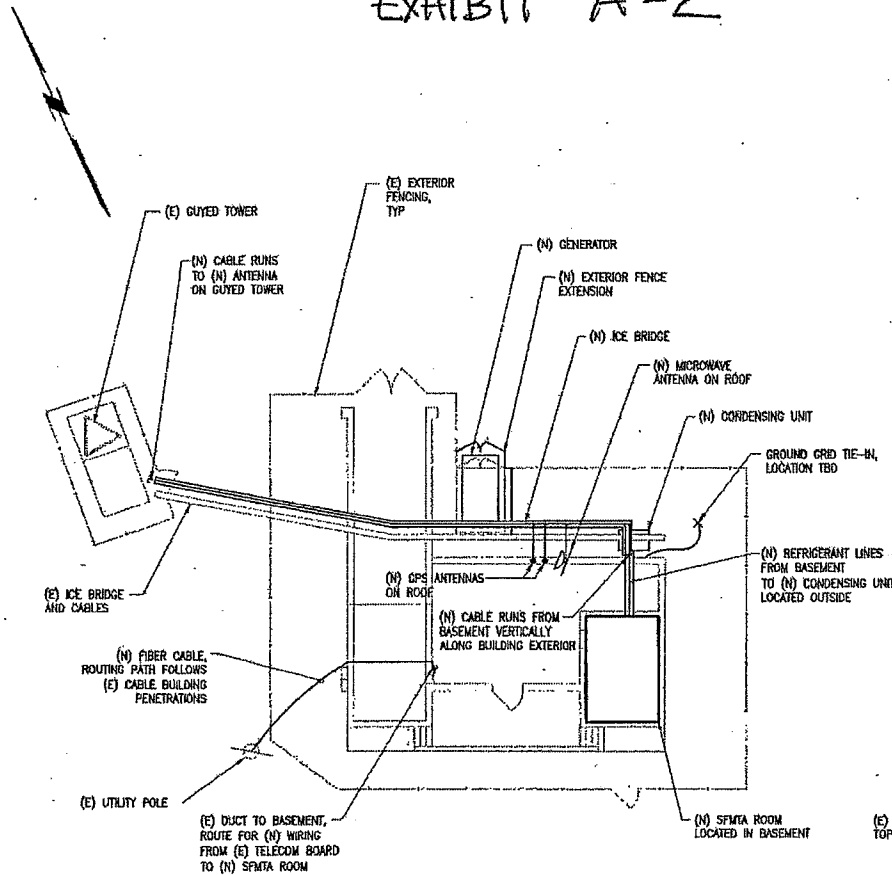
SITE PLAN HTS
