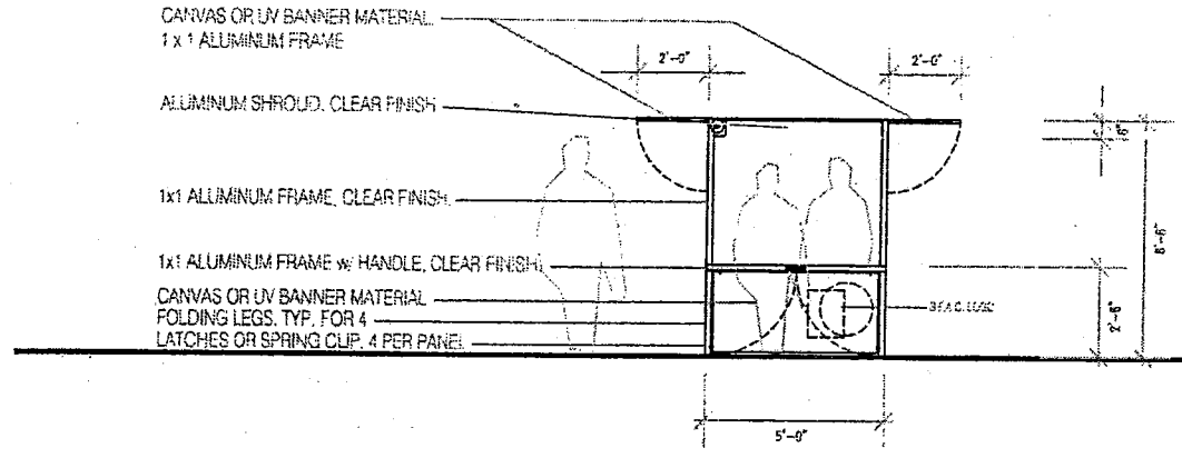
LONG ELEVATION
